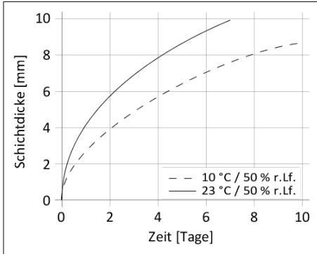
Diagramm 1: Durchhärtageschwindigkeit SikaTack®-MOVE Transportation
