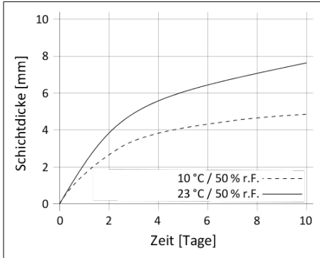
Diagramm 1: Durchhärtengeschwindigkeit Sikaflex®-529 Evolution
