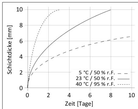
Diagramm 1: Durchhärtegeschwindigkeit von Sikasil® WS-605 S
