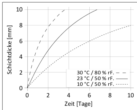
Diagramm 1: Durchhärtengeschwindigkeit Sikaflex®-268
